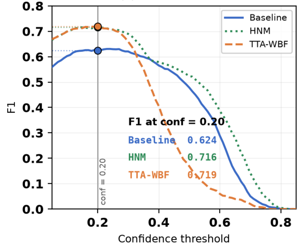
(b) F1 vs confidence
