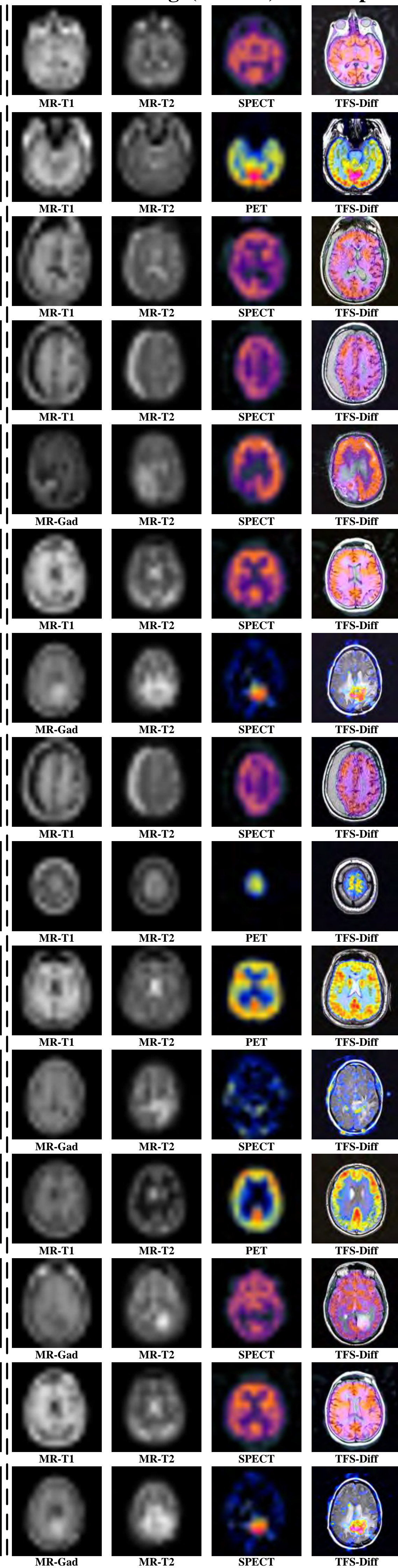
Source Image(Bicubicx8)
